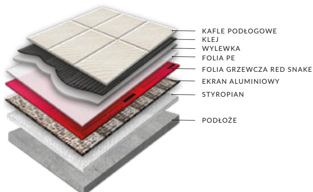
SCHEMAT UŁOŻENIA NA PODŁODZE Z PŁYTKAMI
